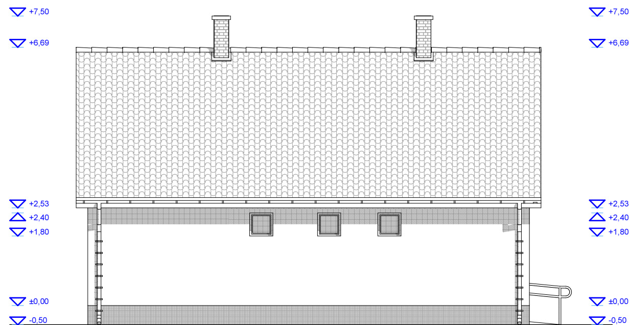
ÉSZAKI HOMLOKZAT
