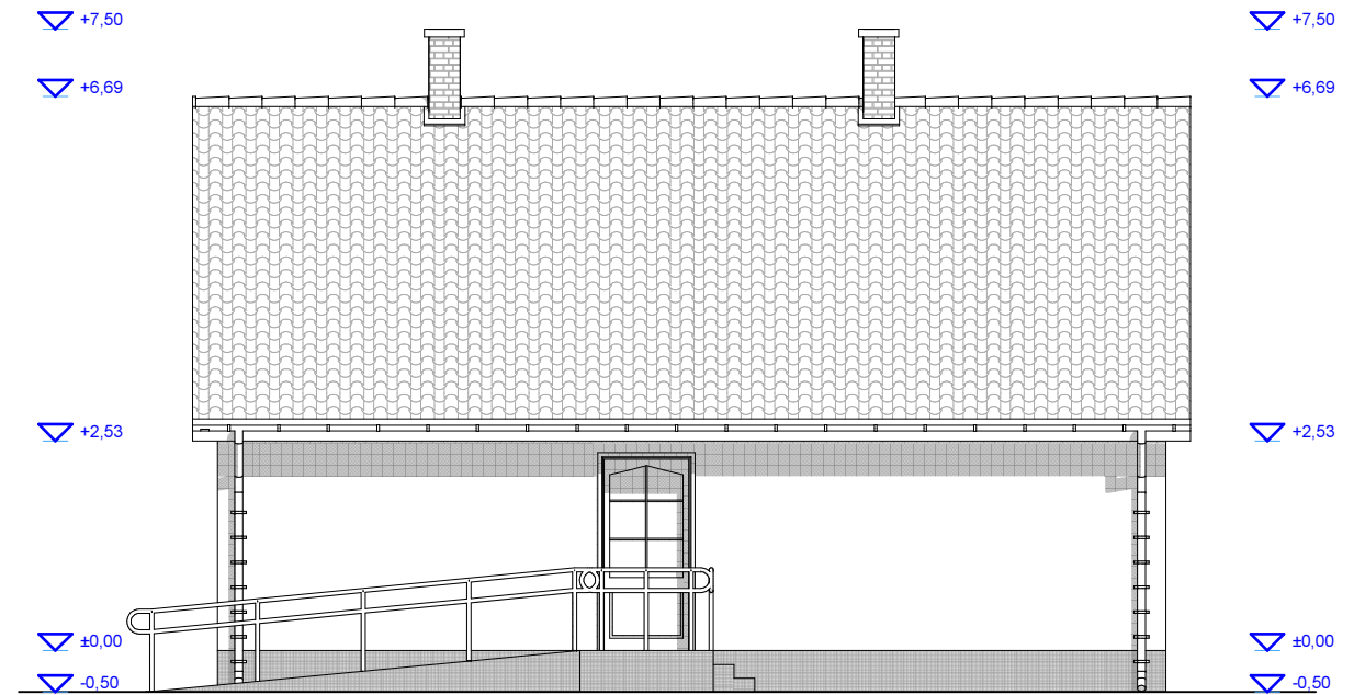
DÉLI HOMLOKZAT
